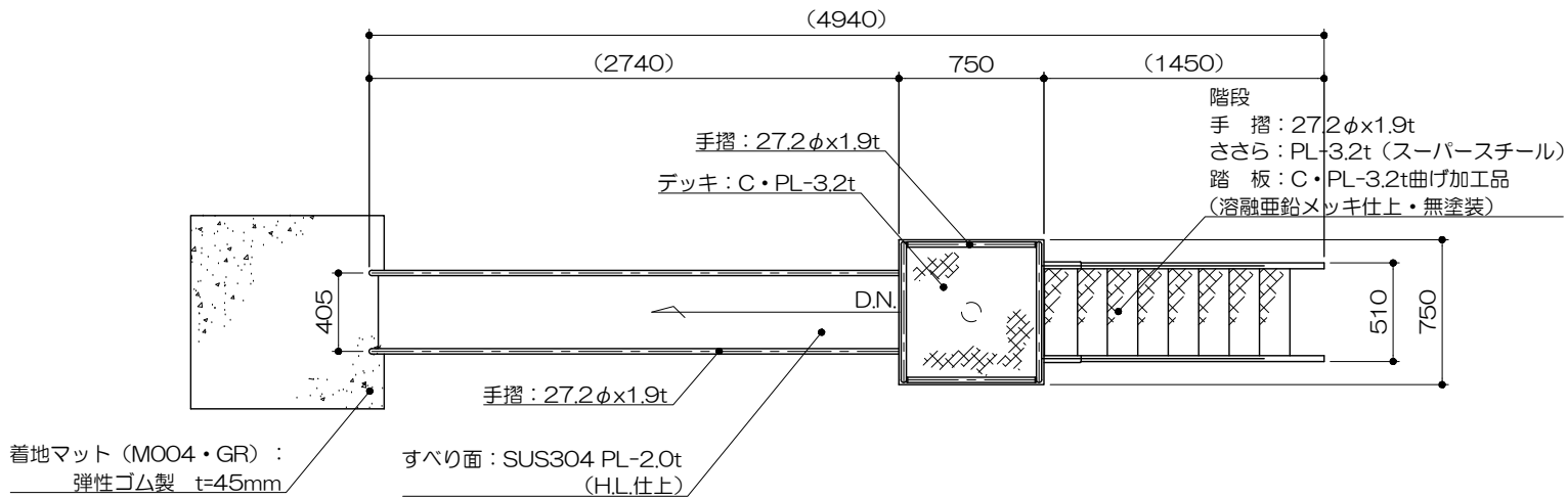
平面図 S= 1 : 40
