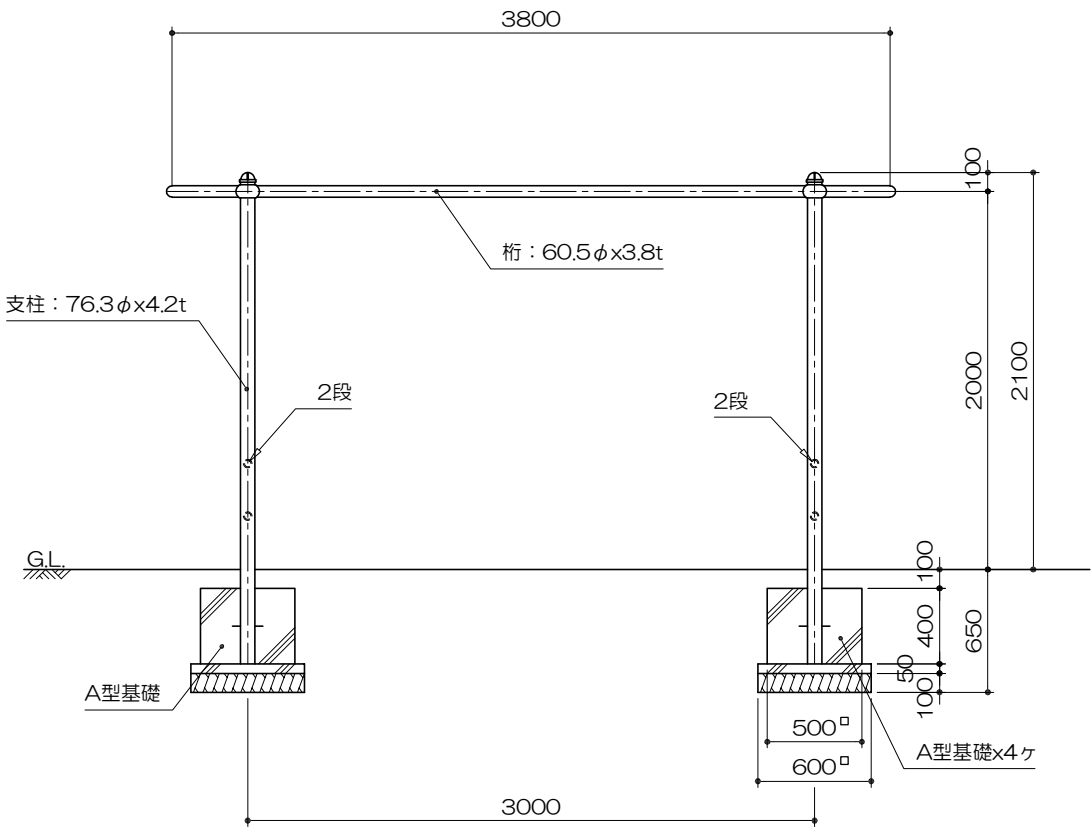
立面図 S= 1 : 40
