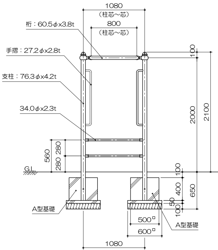
側面図 S= 1 : 40
