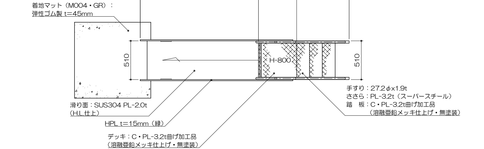
基礎平面図 S= 1 : 30
