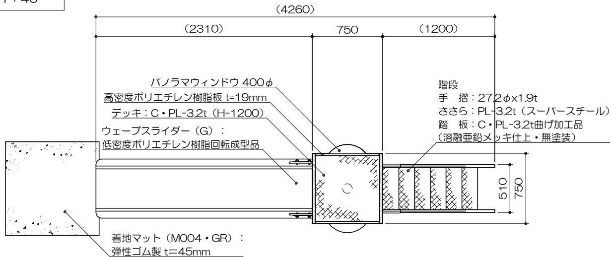
平面図 S= 1 : 40
