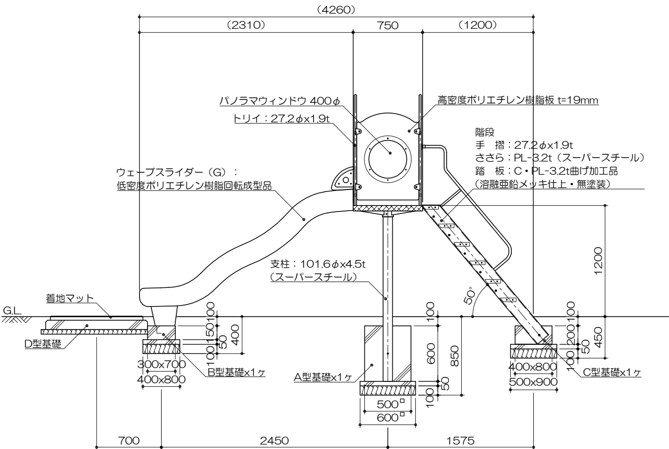
立面図 S= 1 : 40
