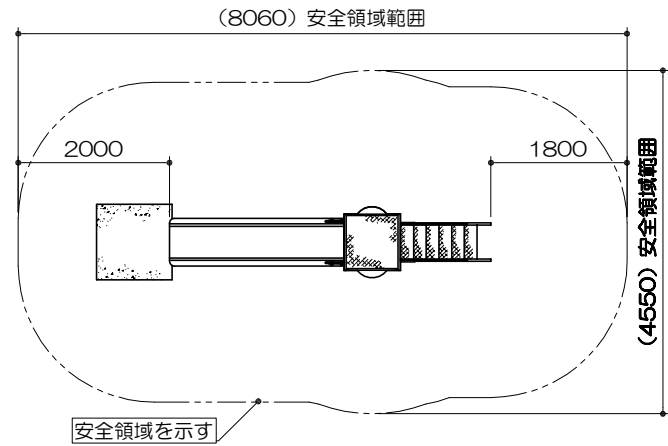
安全領域範囲 S= 1 : 100
