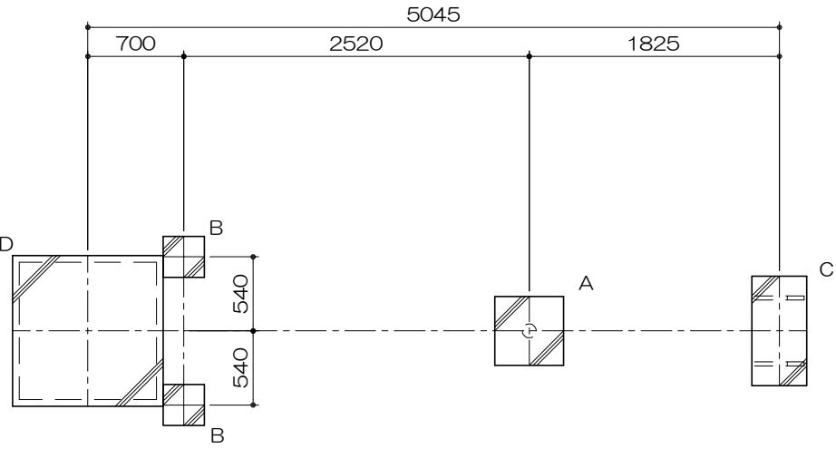
基礎平面図 S= 1 : 50
