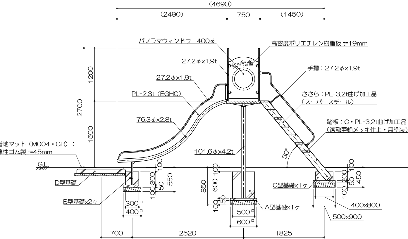
立面図 S= 1 : 50
