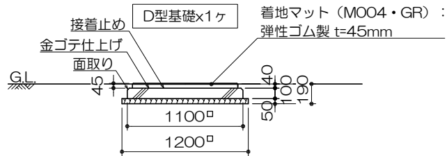
D型基礎詳細図 S= 1 : 50
