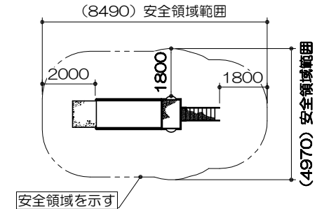
安全領域範囲 S= 1 : 200
