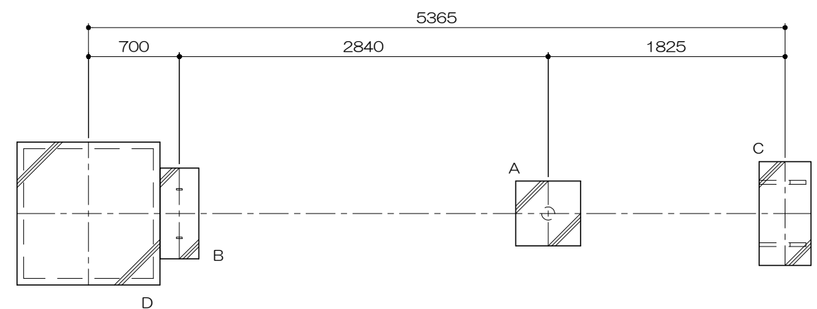
D型基礎詳細図
