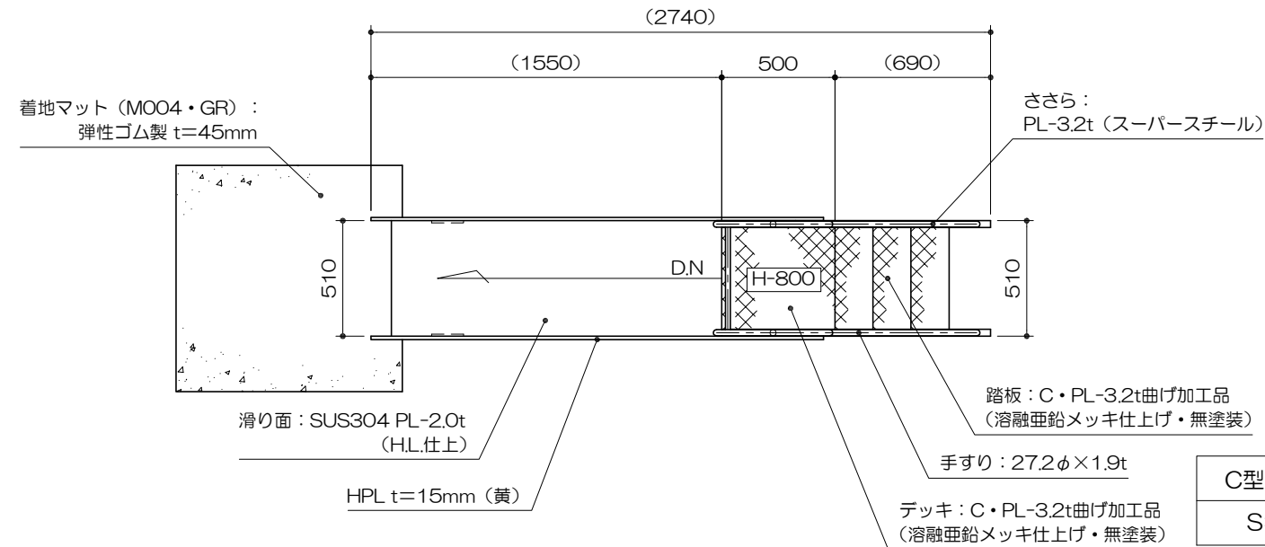
平面図 S=1 : 30
