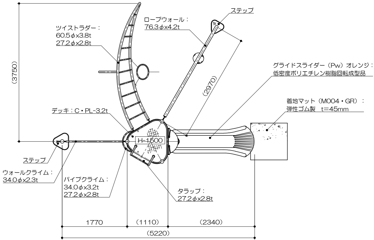
平面図 S= 1 : 60
