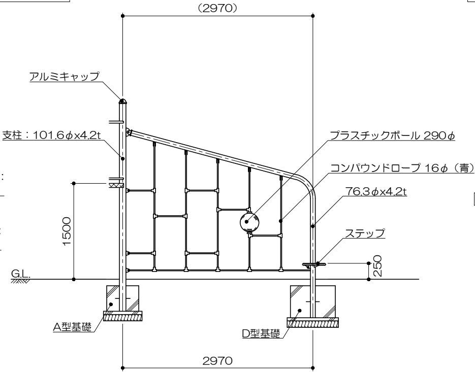
ロープウォール立面図 S= 1 : 60
