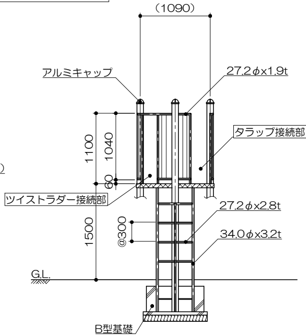
パイプクライム立面図 S= 1 : 60
