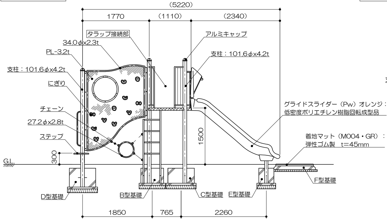
立面図 S= 1 : 60
