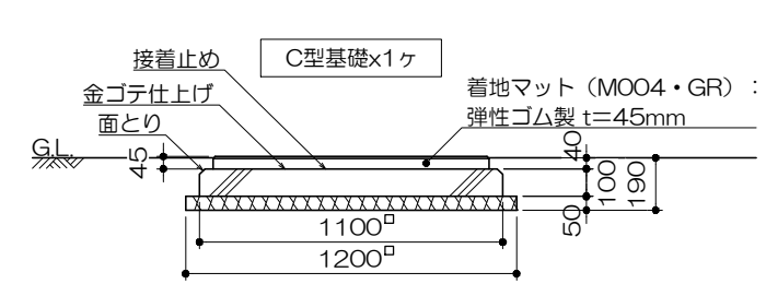
C型基礎詳細図 S= 1 : 30
