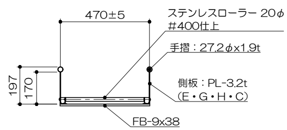
a-a断面図 S= 1 : 20
