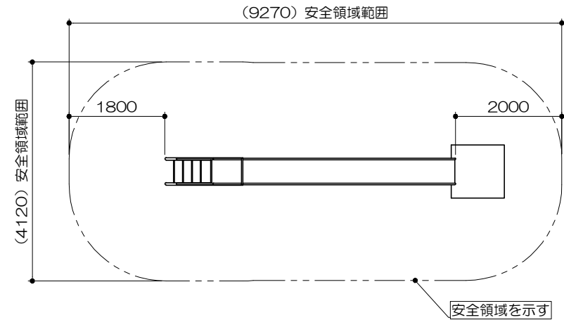
安全領域範囲 S= 1 : 100
