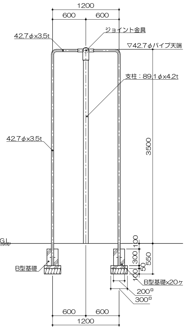
側面図 S= 1 : 40
