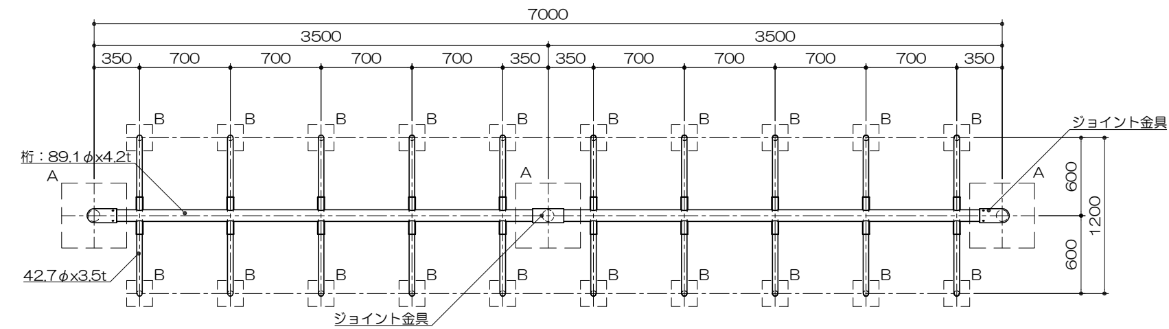
平面図 S= 1 : 40
