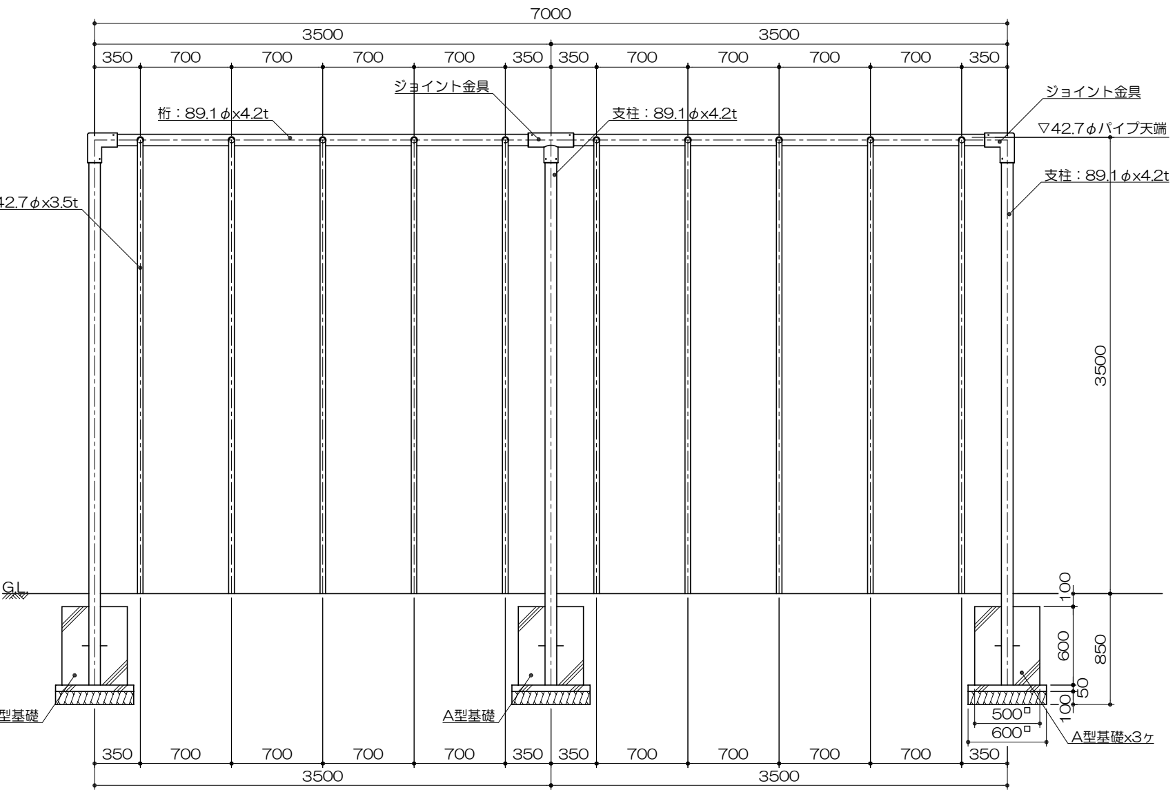
立面図 S= 1 : 40
