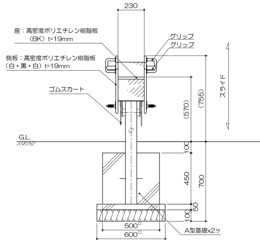
側面図 S= 1 : 20
