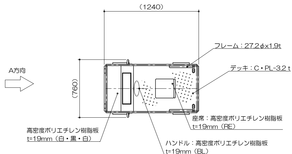
平面図 S=1 : 30
