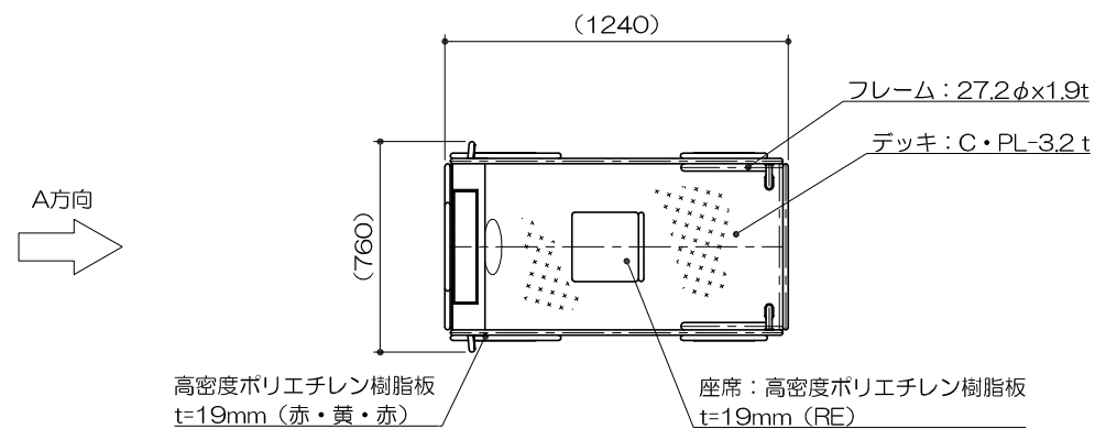
平面図 S=1 : 30
