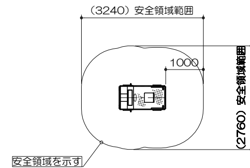
安全領域範囲 S=1:100
