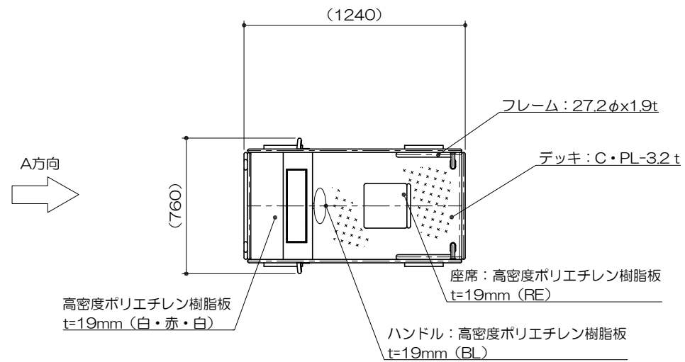
平面図 S=1:30
