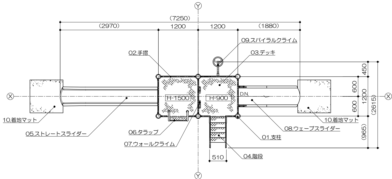
平面図 S= 1 : 60
