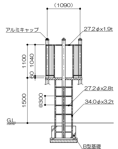
パイプクライム立面図 S= 1 : 60
