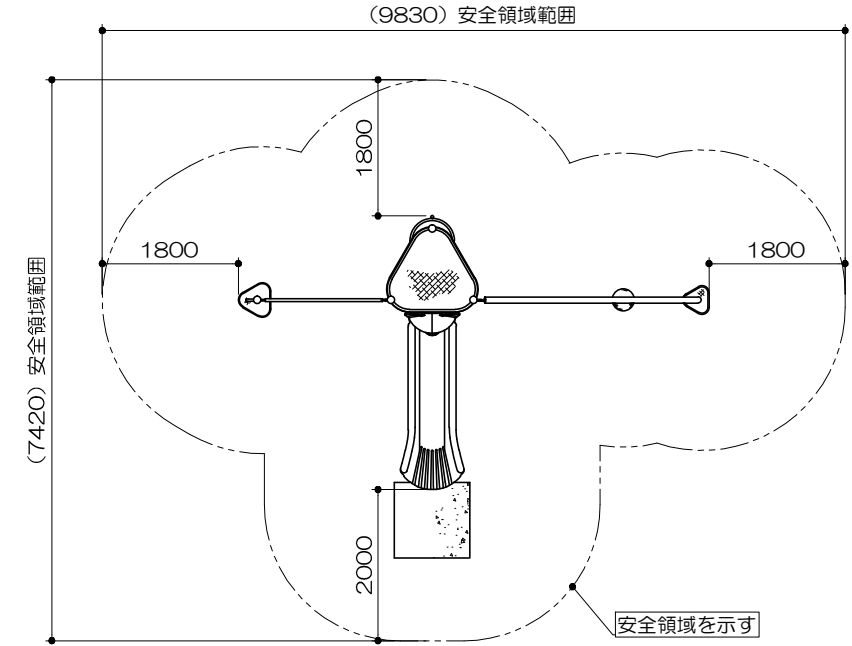
安全領域範囲 S= 1 : 100
