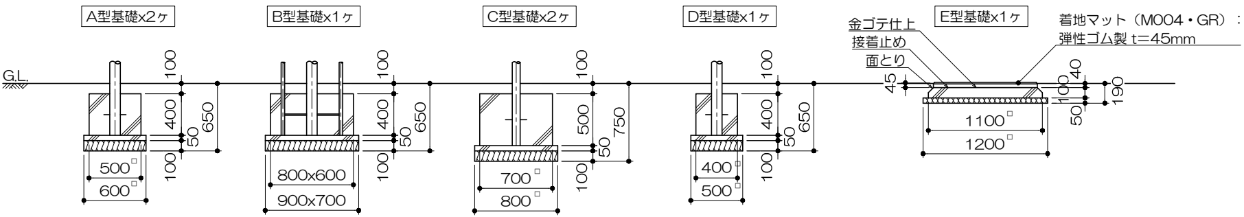
基礎リスト S= 1 : 50
