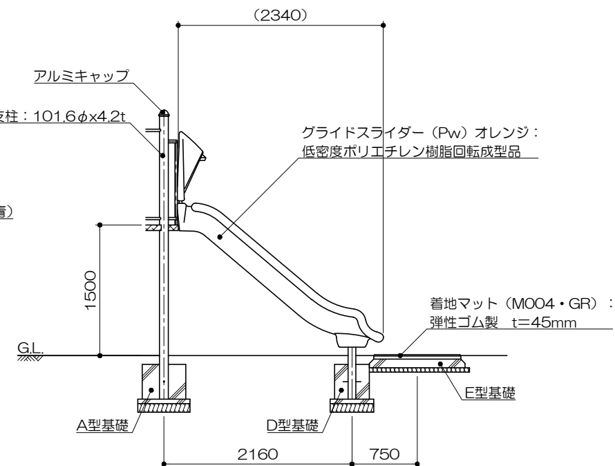
グライドスライダー立面図 S= 1 : 60
