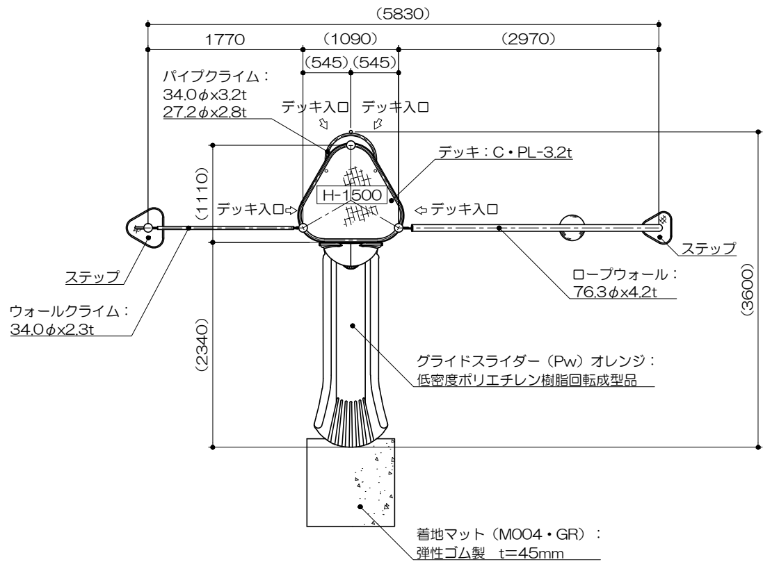
平面図 S= 1 : 60
