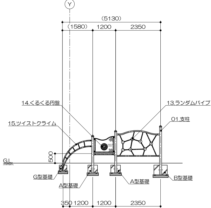
立面図 S= 1 : 100
