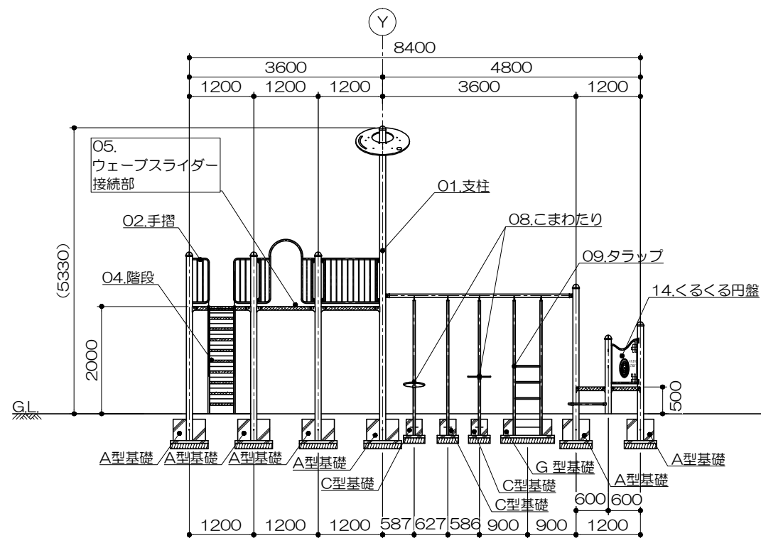
b-b展開図
