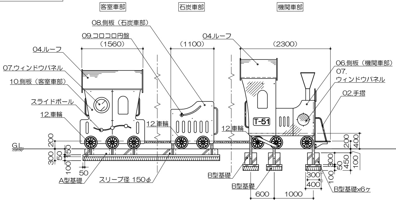
立面図 S= 1 : 60
