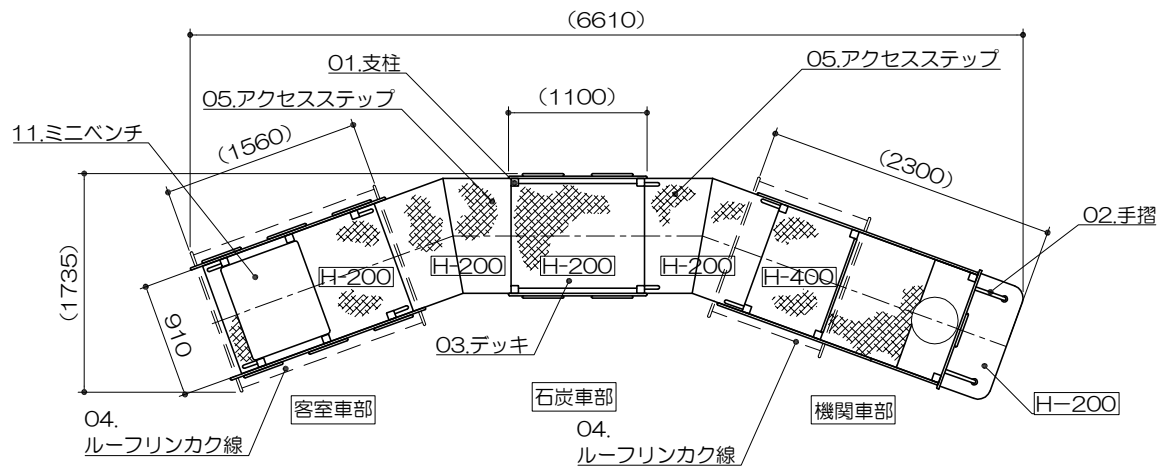
平面図 S= 1 : 60
