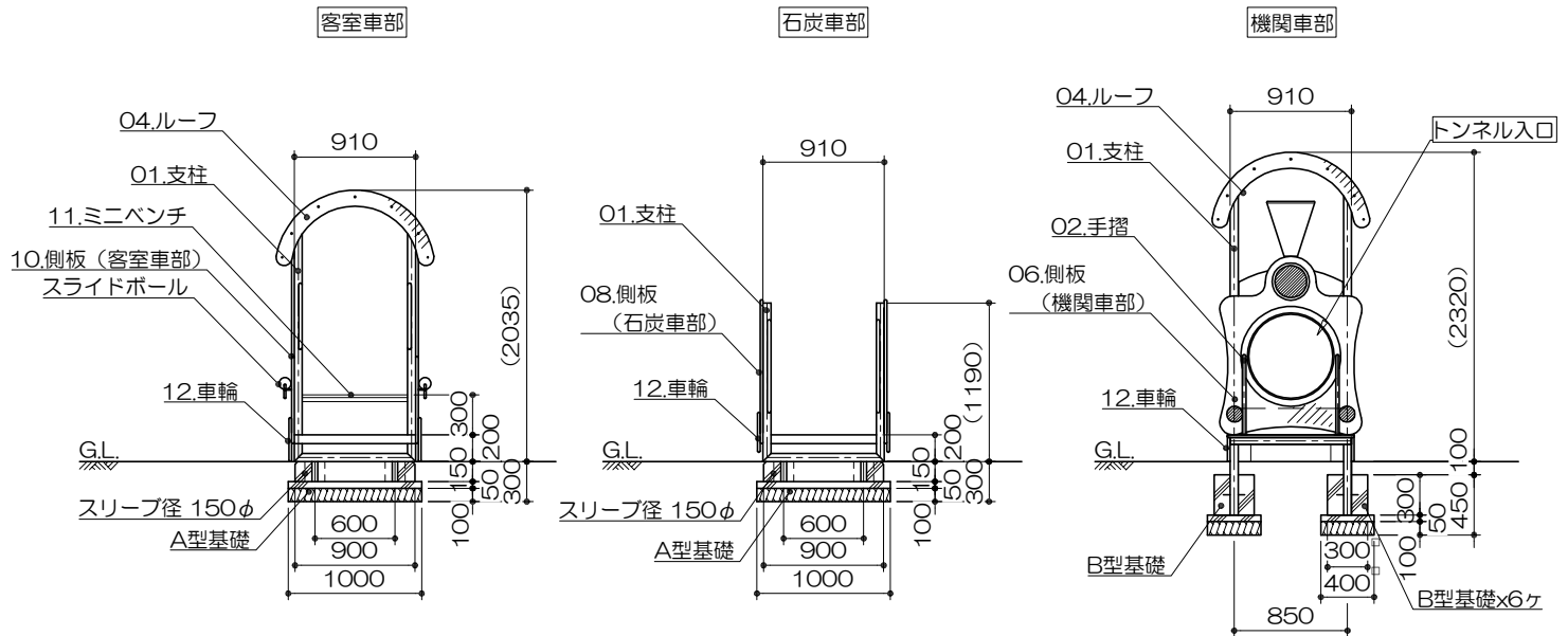
正面図 S= 1 : 60
