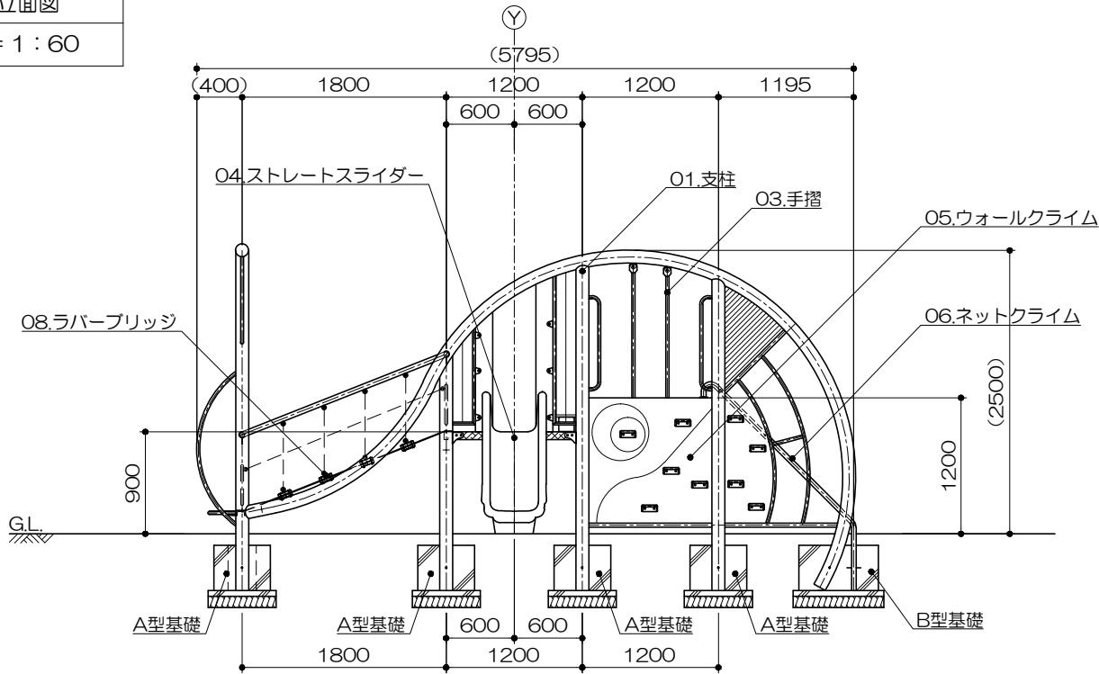
側面図 S= 1 : 60
