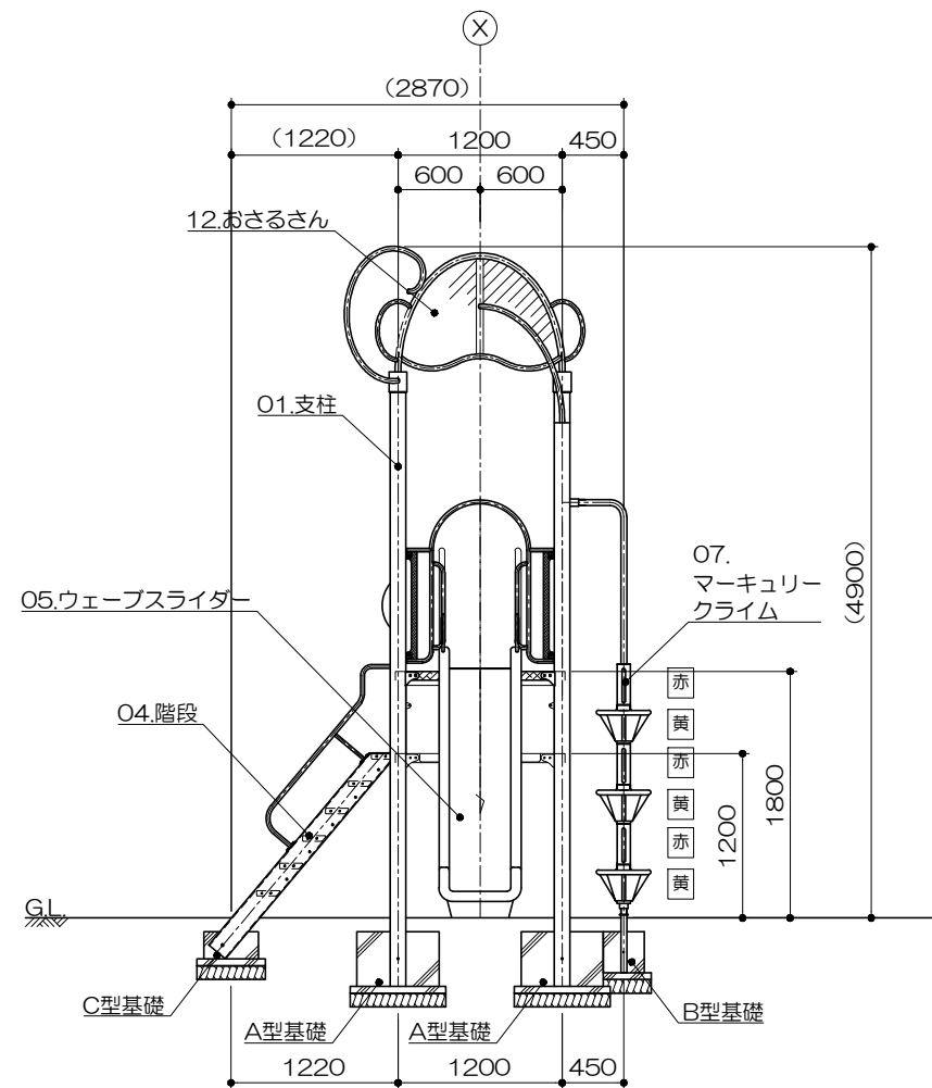
側面図 S= 1 : 60
