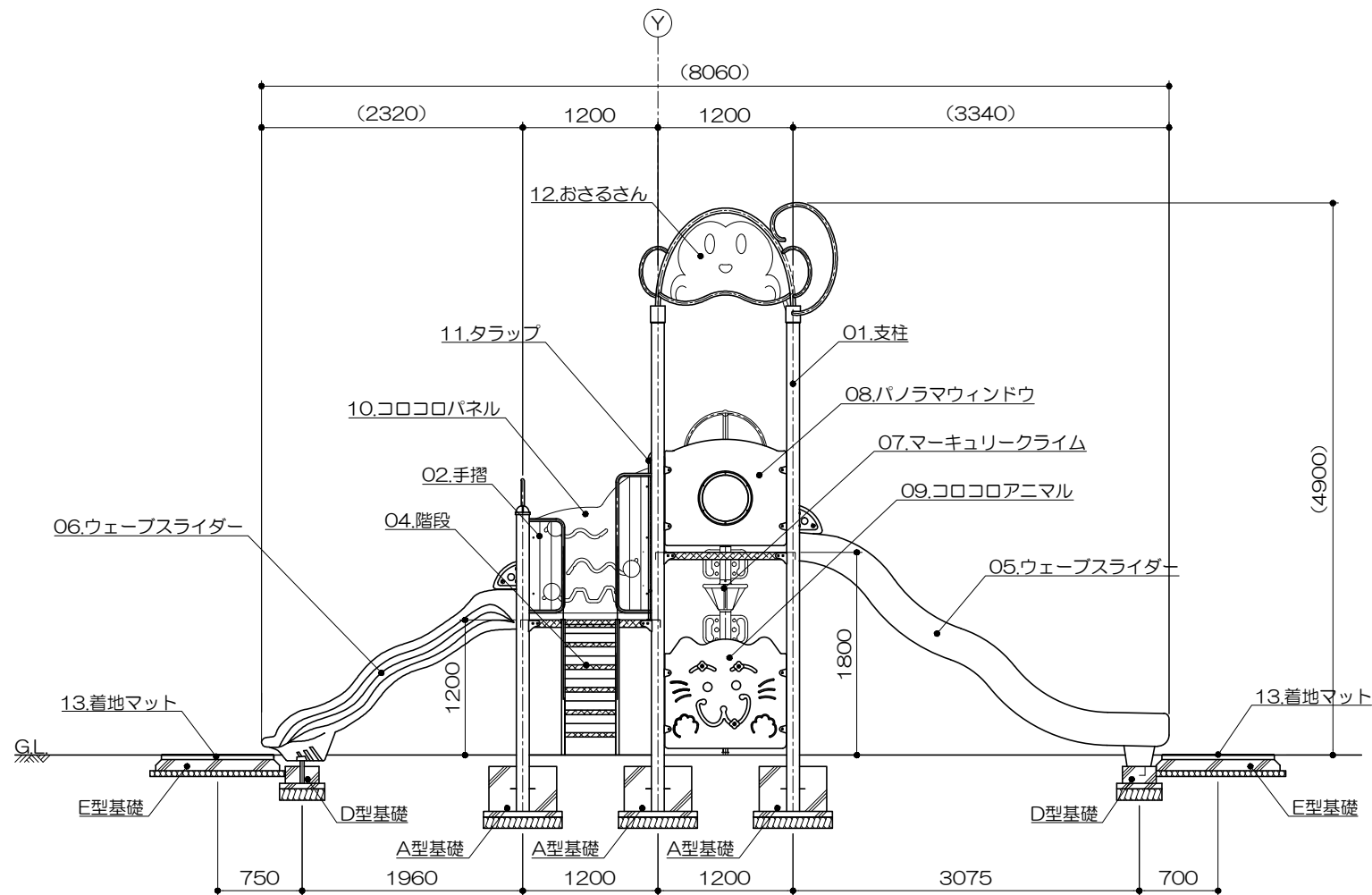
立面図 S= 1 : 60
