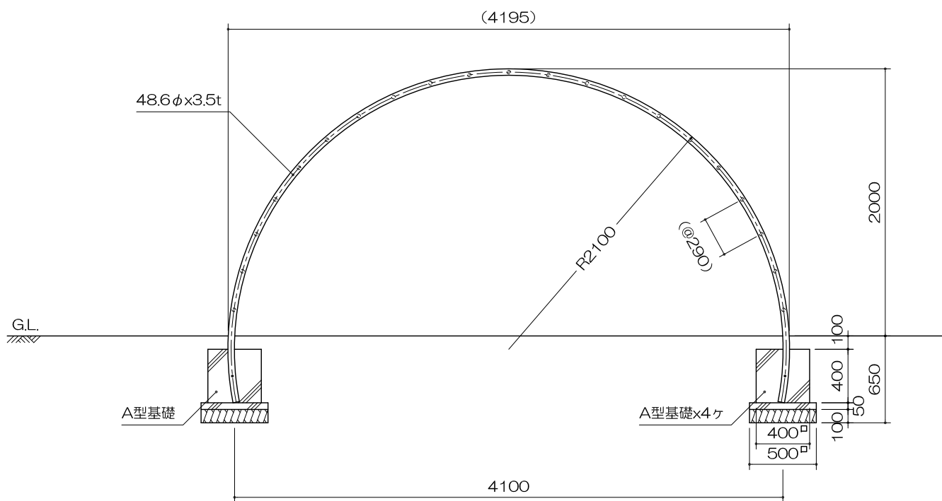
立面図 S= 1 : 40
