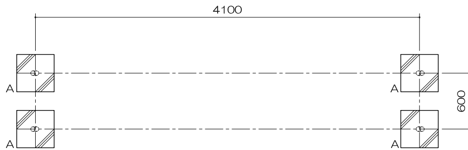
基礎平面図 S= 1 : 40
