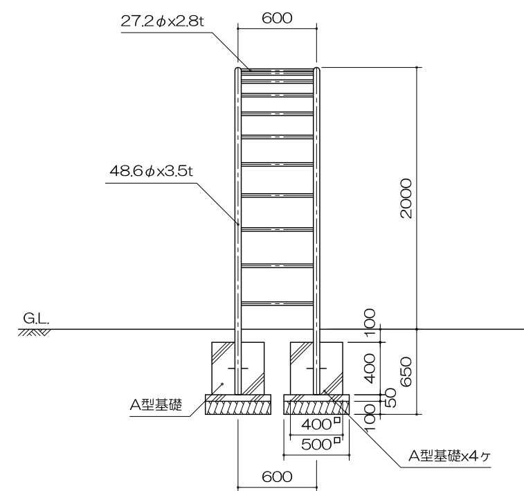
側面図 S= 1 : 40
