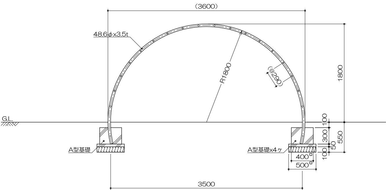
立面図 S= 1 : 40
