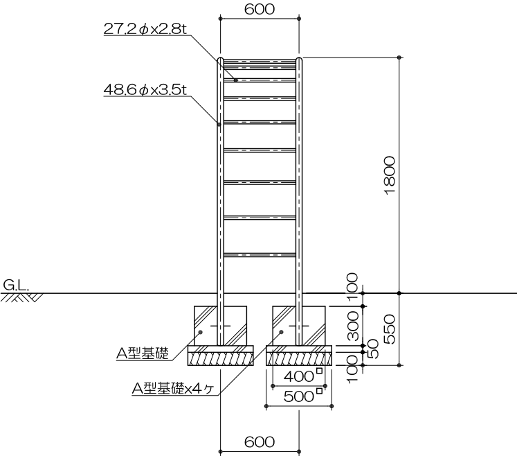
側面図 S= 1 : 40
