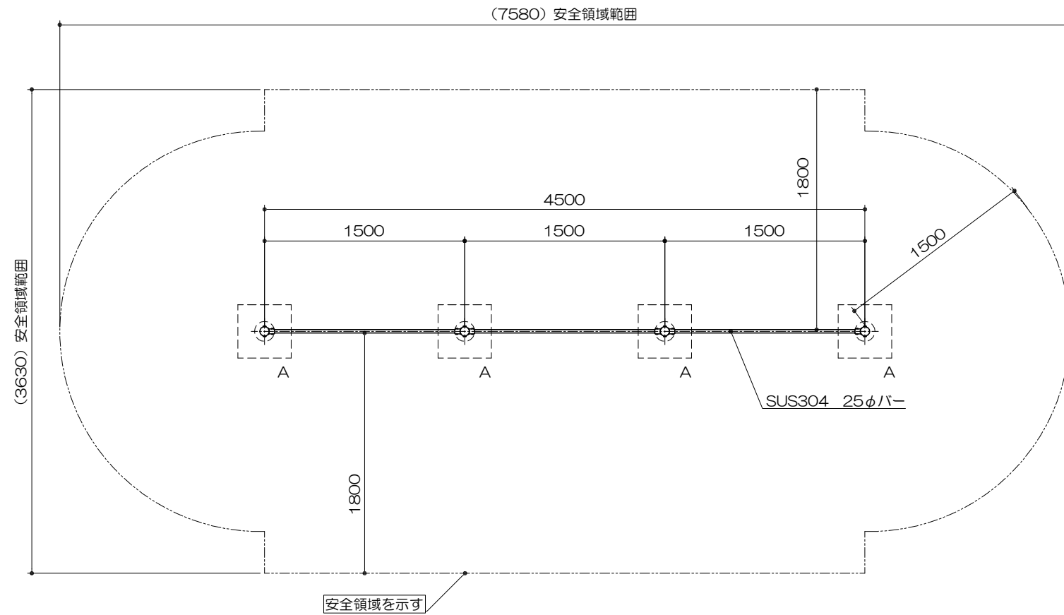
平面図 S= 1 : 40
