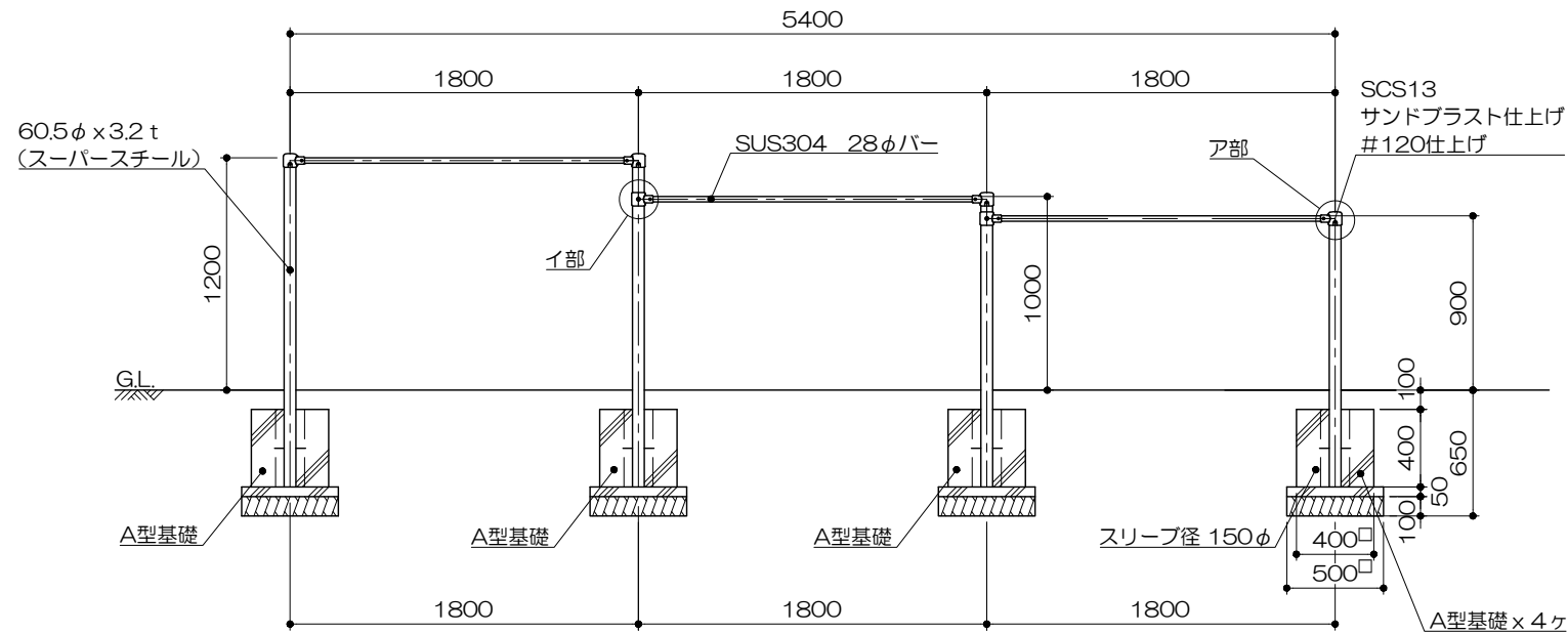
立面図 S= 1 : 40
