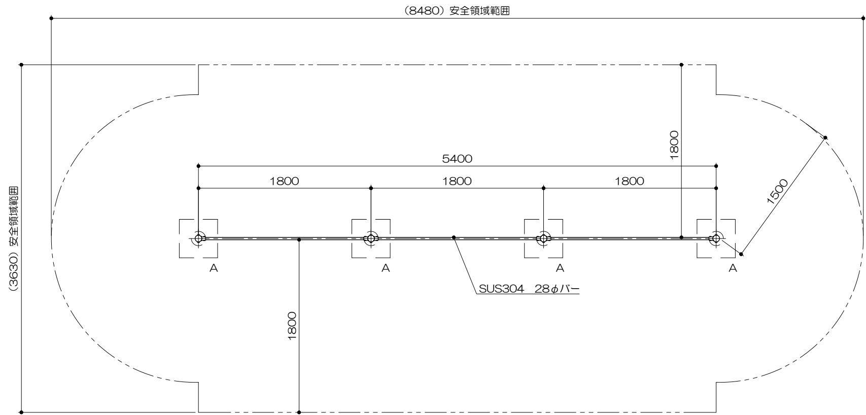
平面図 S= 1 : 40
