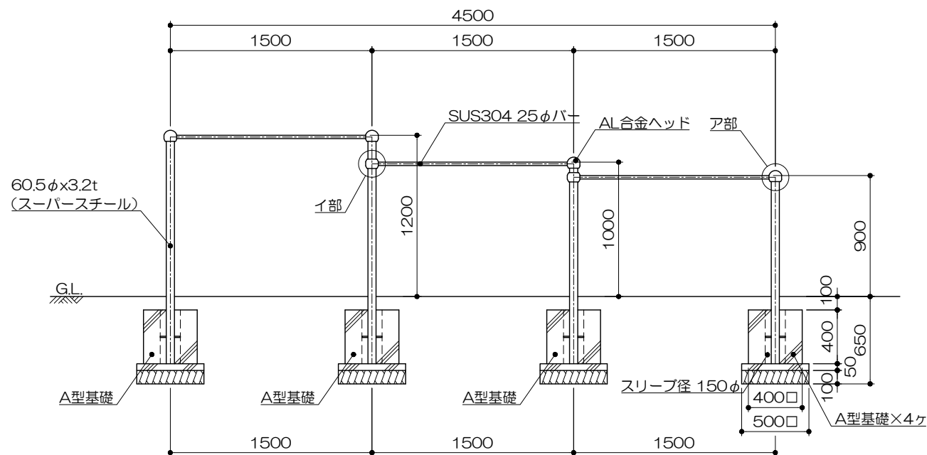
立面図 S= 1 : 40
