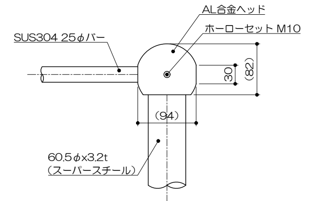
ア部詳細図 S= 1 : 6
