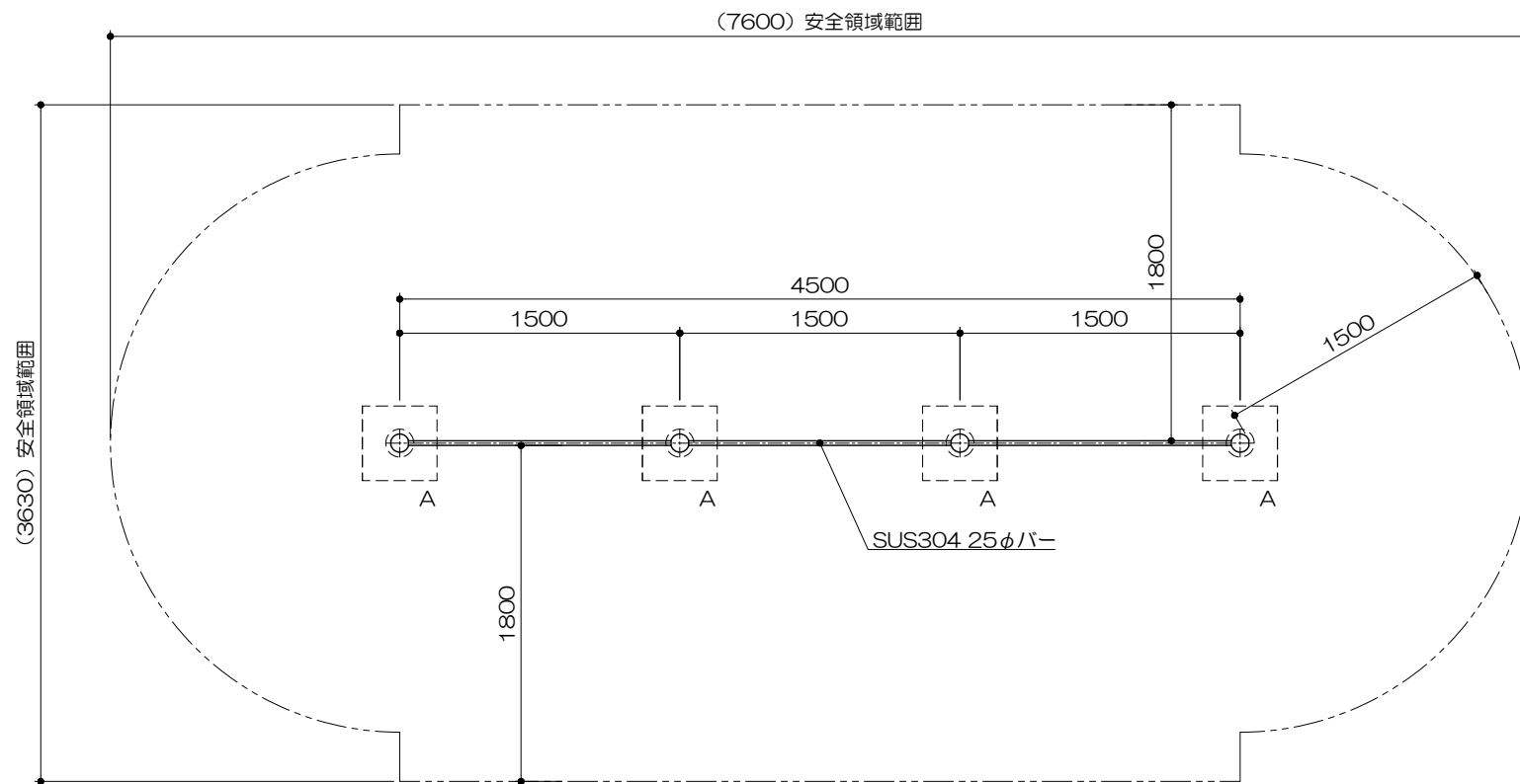
平面図 S= 1 : 40
