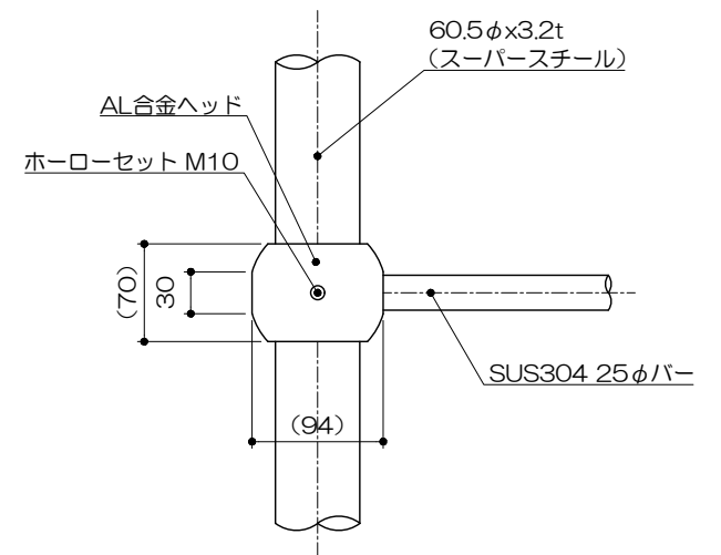
イ部詳細図 S= 1 : 6
