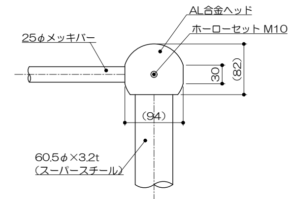
イ部詳細図
