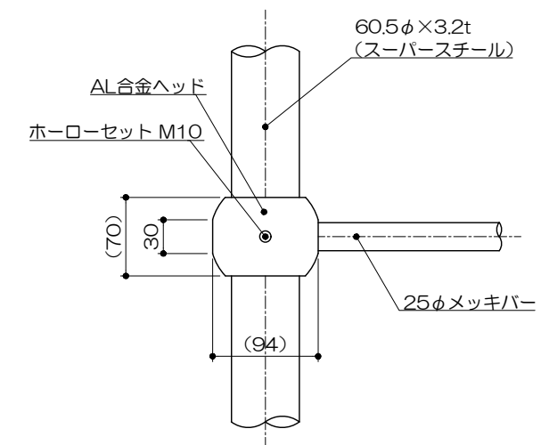
イ部詳細図
