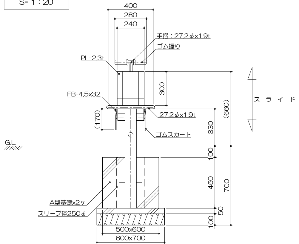
側面図 S= 1 : 20
