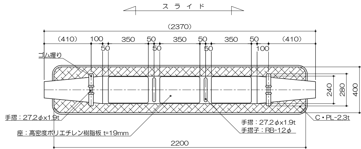
平面図 S= 1 : 20
