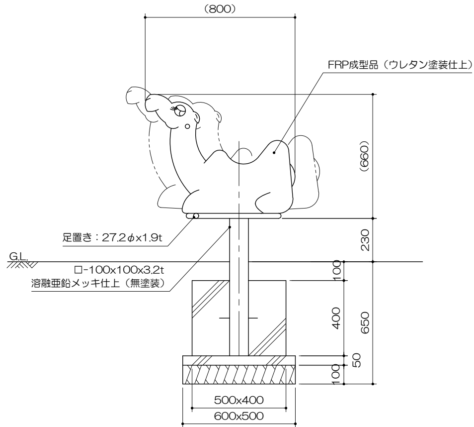
立面図 S= 1 : 20
