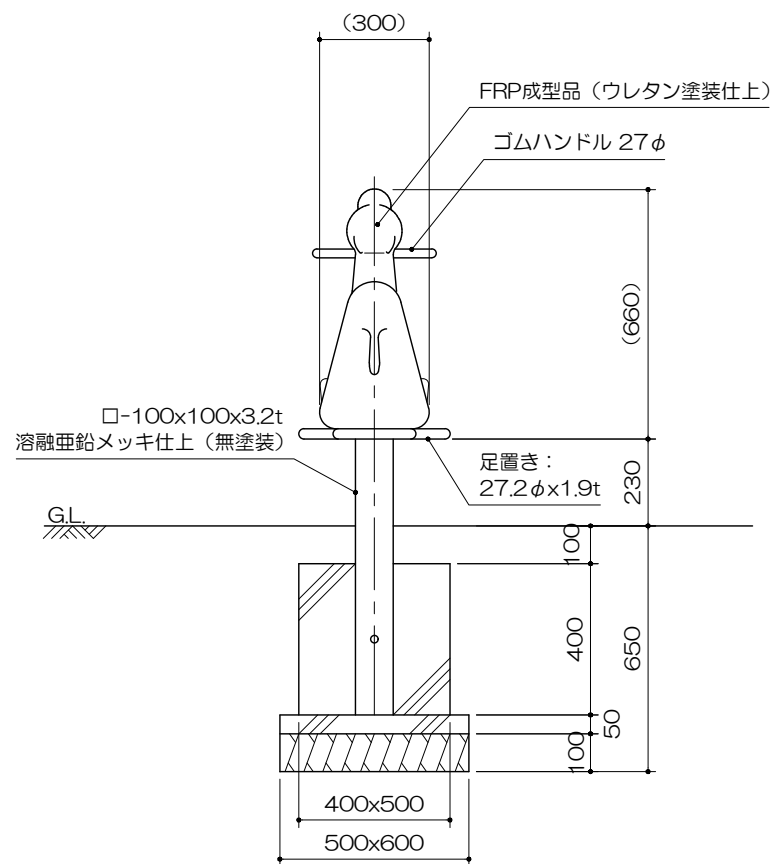
側面図 S= 1 : 20
