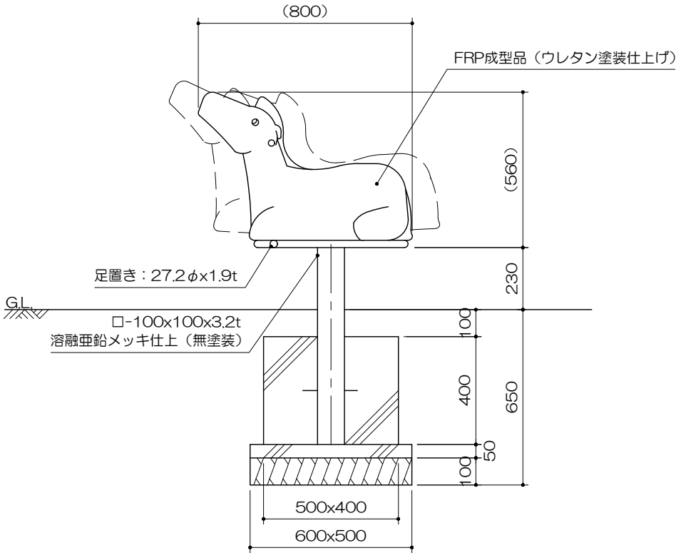
立面図 S= 1 : 20
