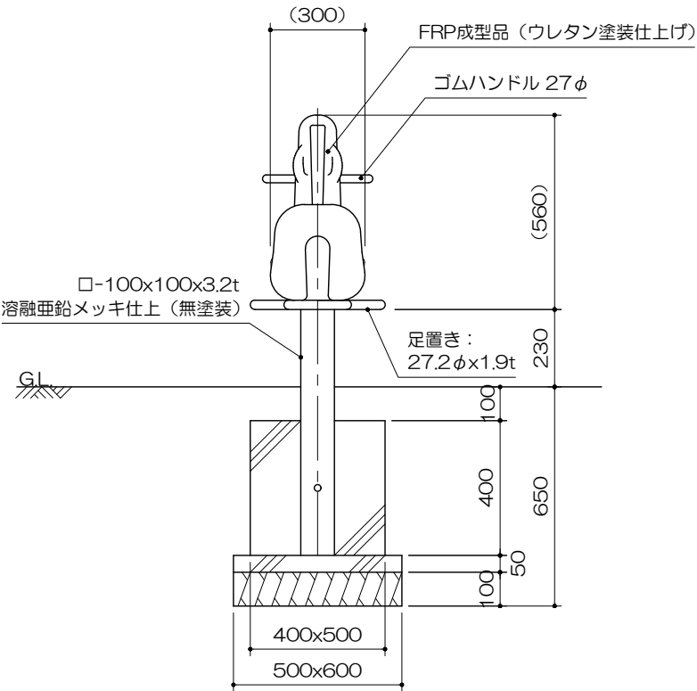
側面図 S= 1 : 20
