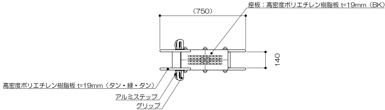
平面図 S= 1 : 20
