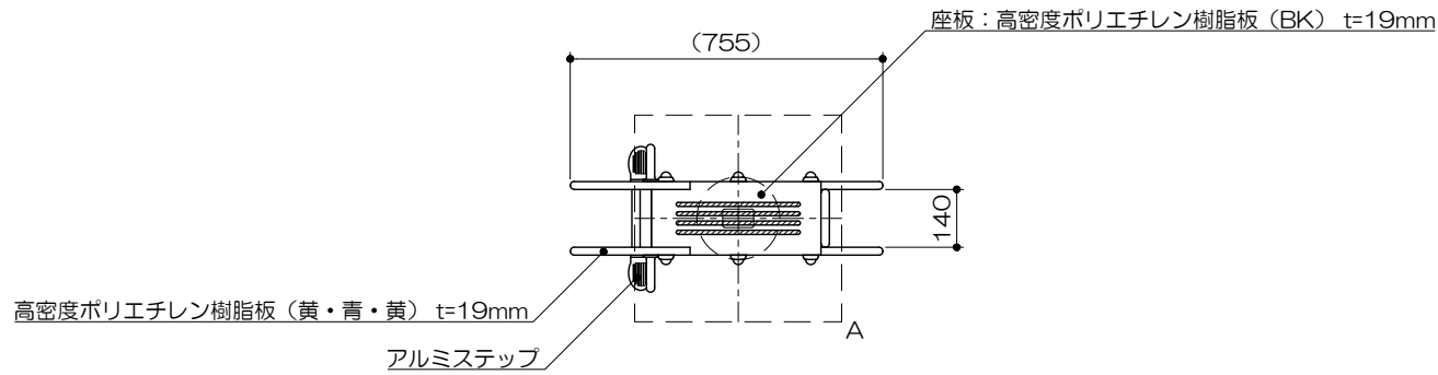
平面図 S= 1 : 20
