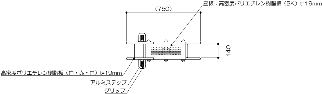
平面図 S= 1 : 20
