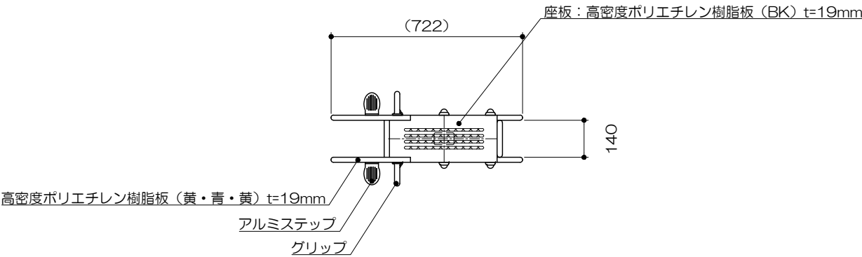
平面図 S= 1 : 20
