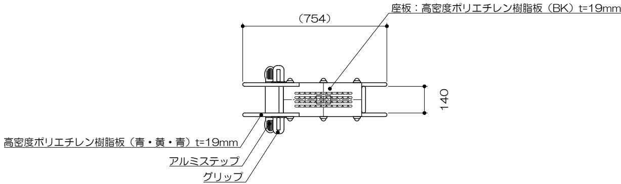
平面図 S= 1 : 20
