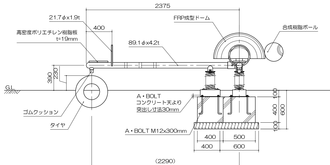
S= 1 : 30
