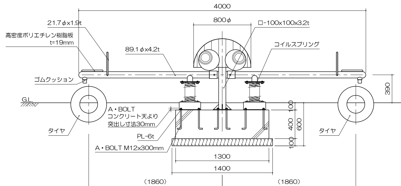
S= 1 : 30
