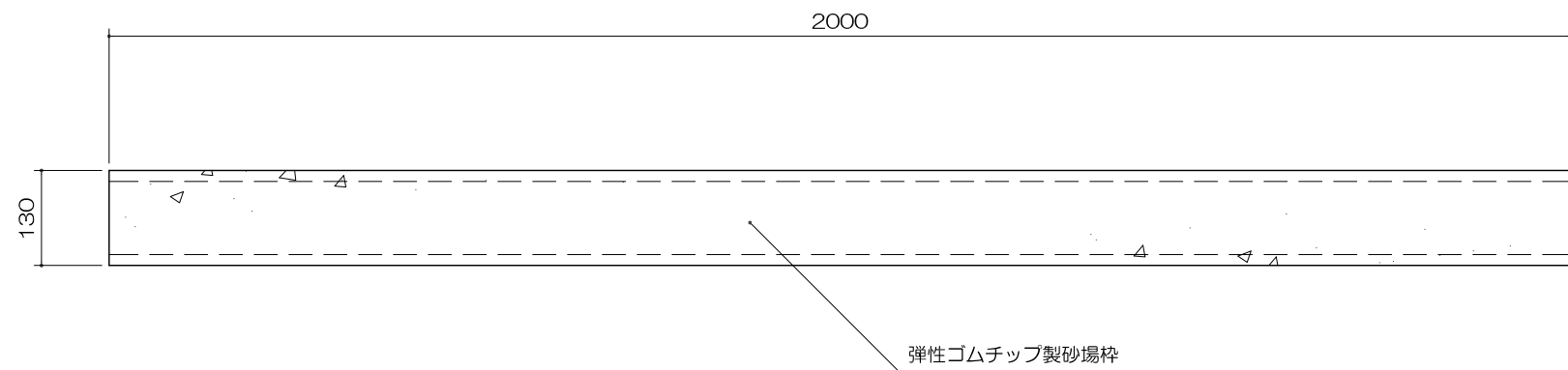
平面図 S= 1 : 10
