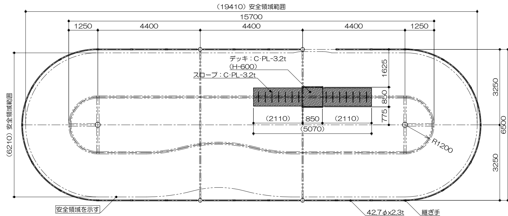
平面図 S= 1 : 100
