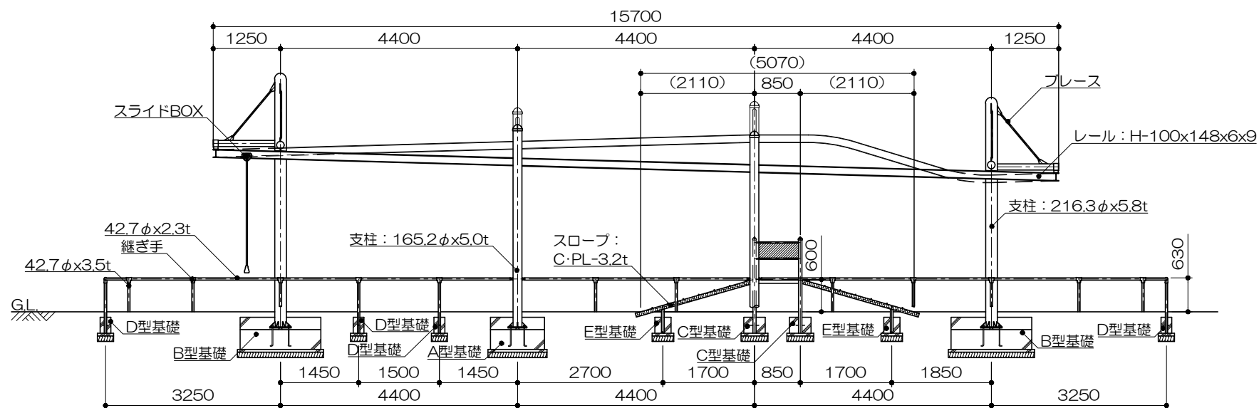
立面図 S= 1 : 100
