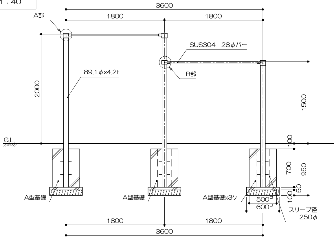
立面図 S= 1 : 40
