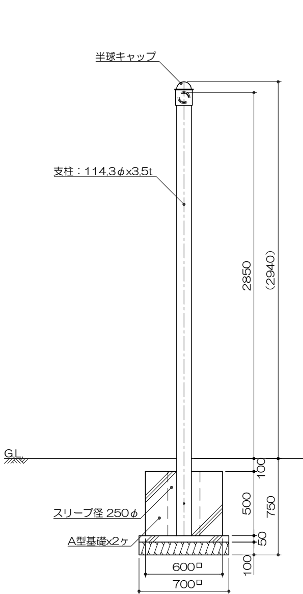
側面図 S= 1 : 30
