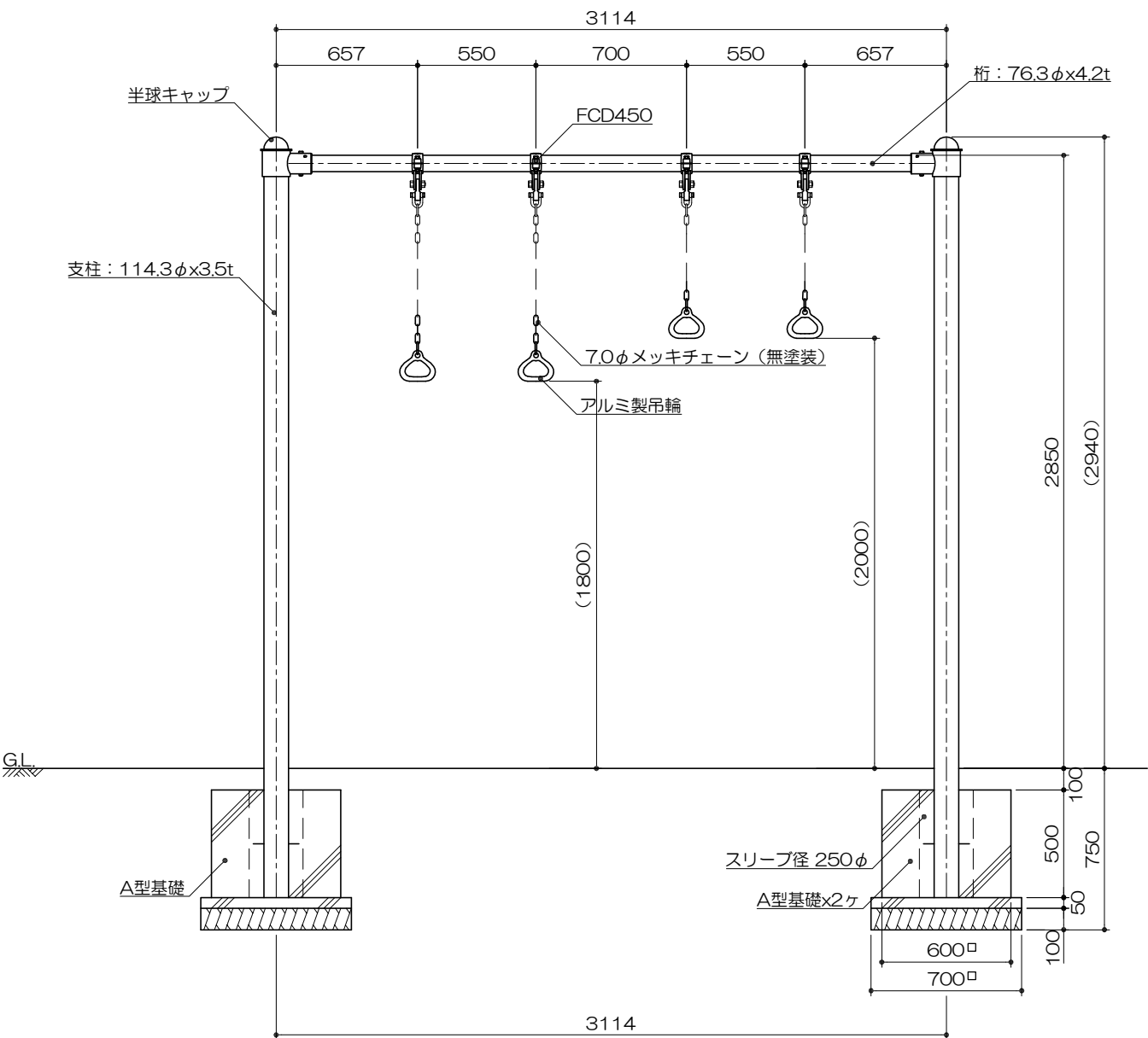
立面図 S= 1 : 30
