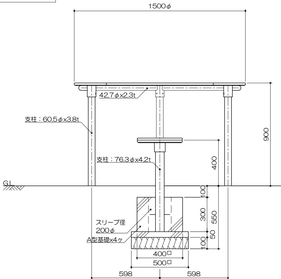
立面図 S= 1 : 20
