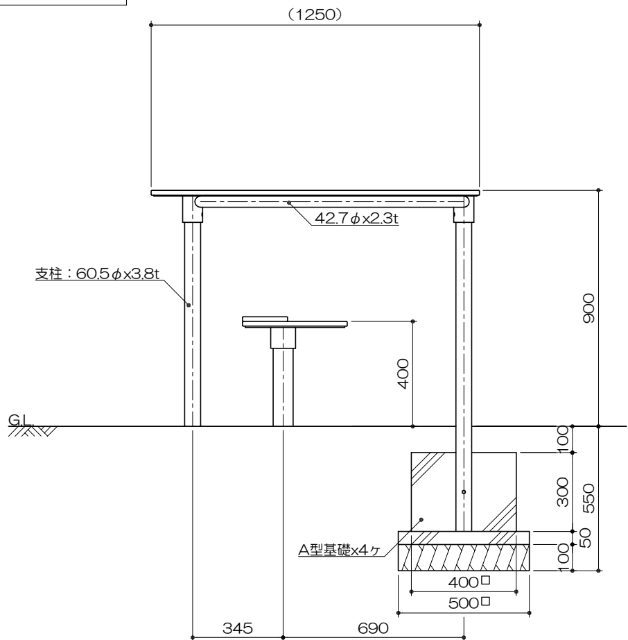
側面図 S= 1 : 20
