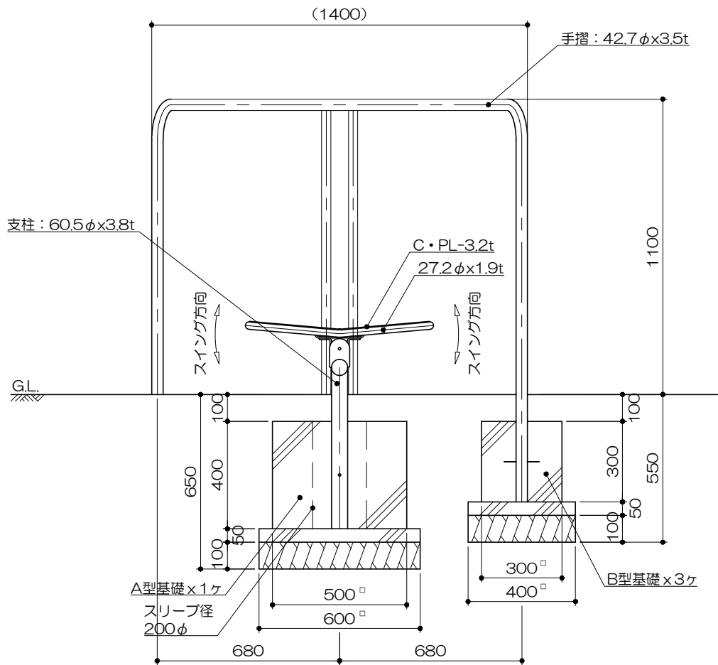
立面図 S= 1 : 20
