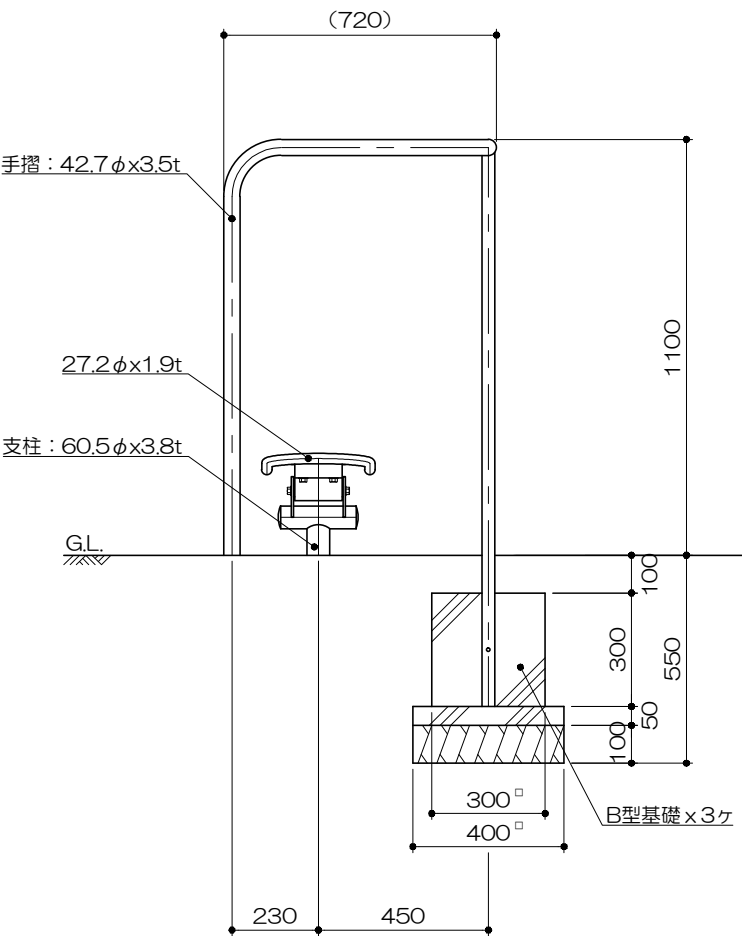
側面図 S= 1 : 20
