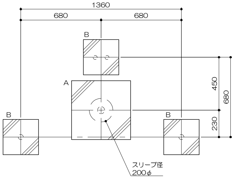
基礎平面図 S= 1 : 20
