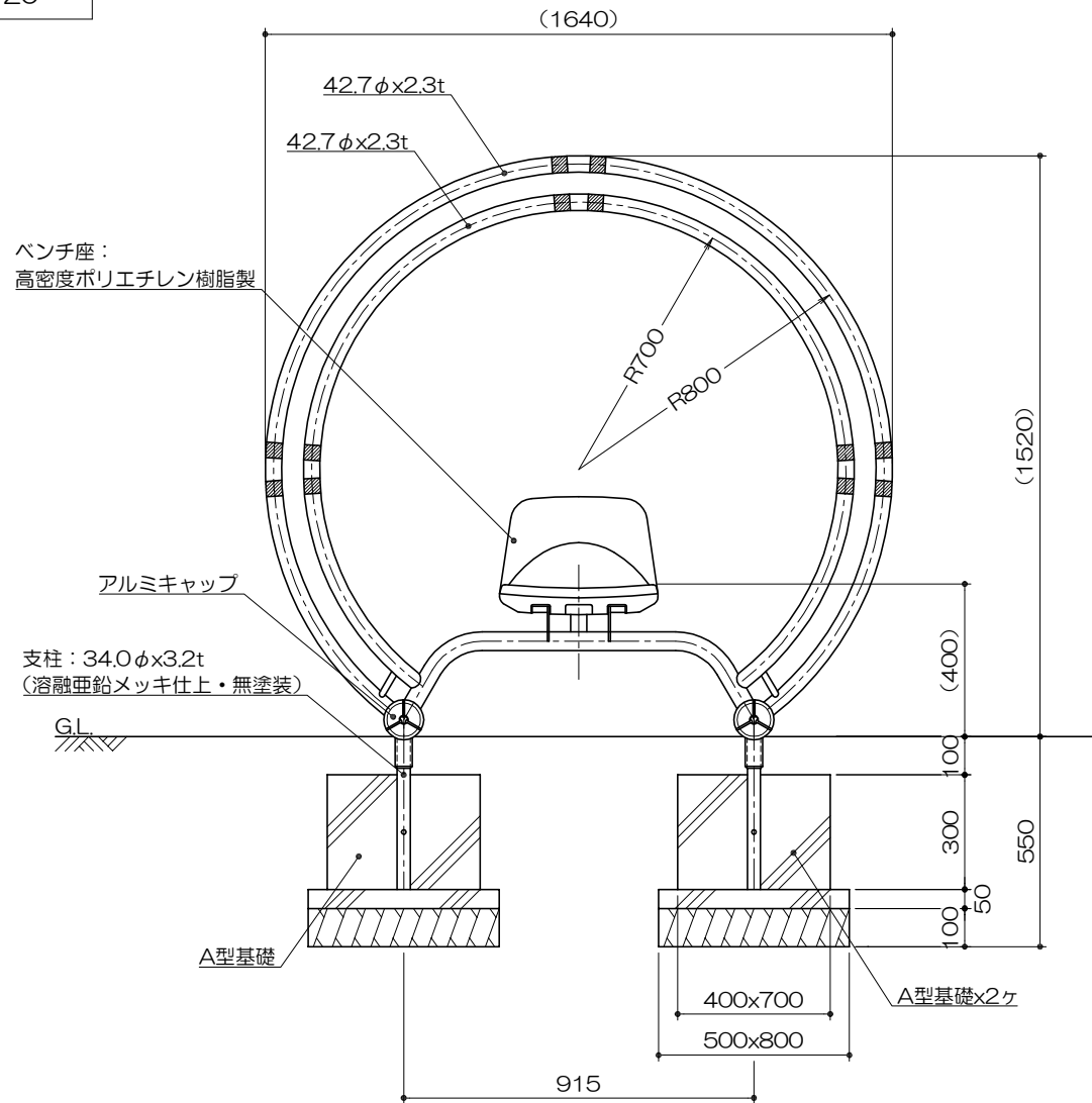
立面図 S= 1 : 20
