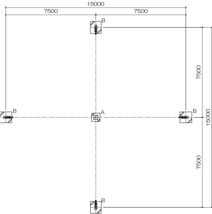
基礎リスト S= 1 : 50
