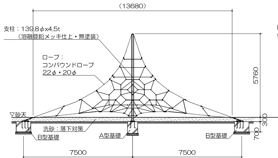
立面図 S= 1 : 150
