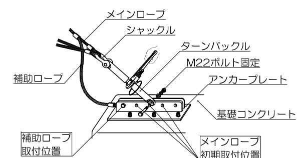
ロープ接続部詳細図
