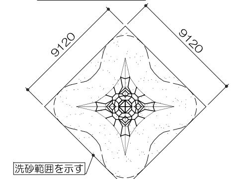
洗砂範囲 S= 1 : 300
