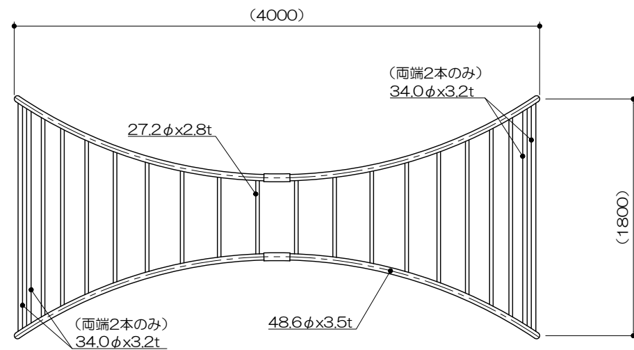
平面図 S= 1 : 40
