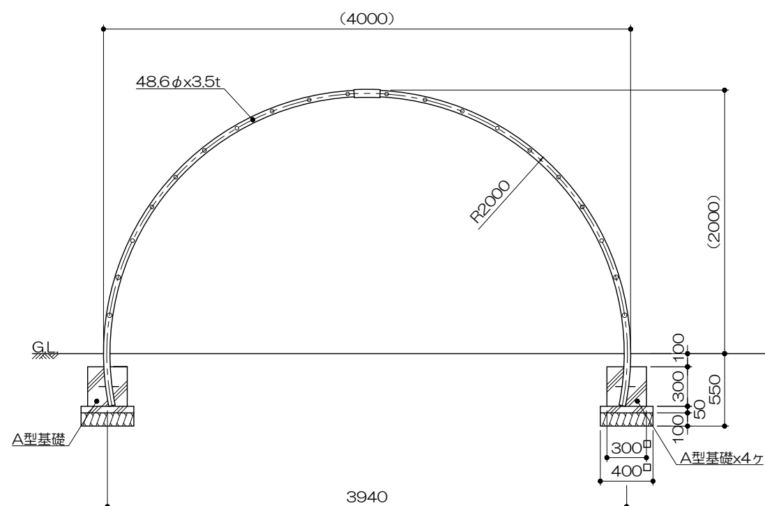
立面図 S= 1 : 40
