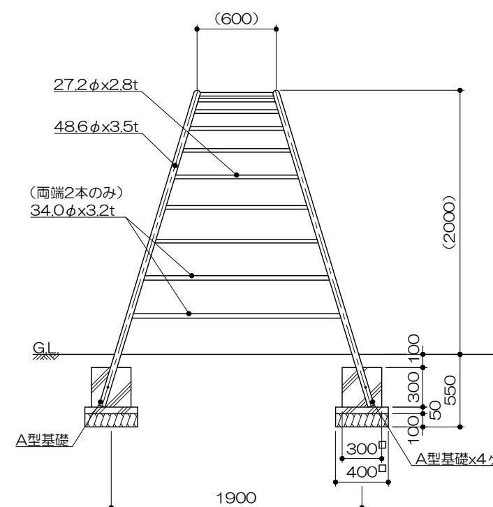
側面図 S= 1 : 40
