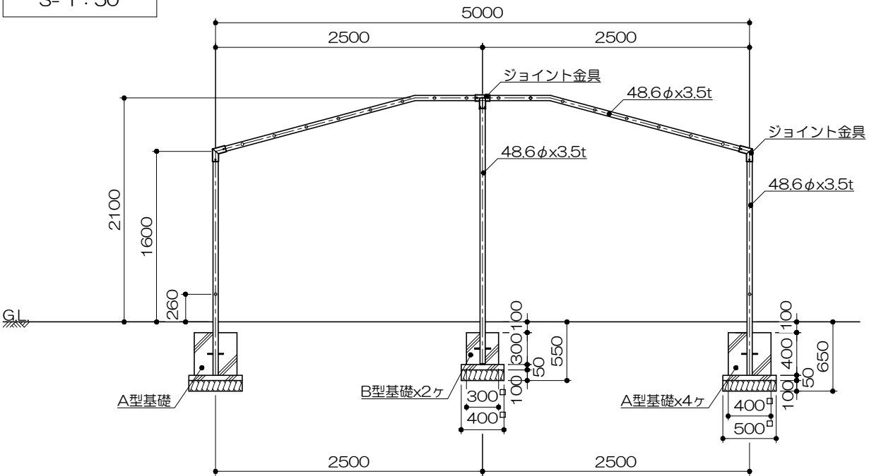
立面図 S= 1 : 50
