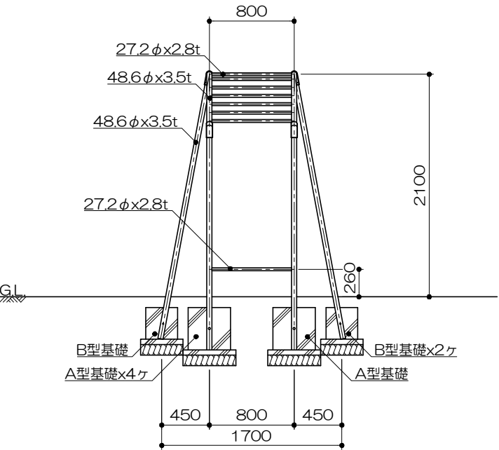
側面図 S= 1 : 50
