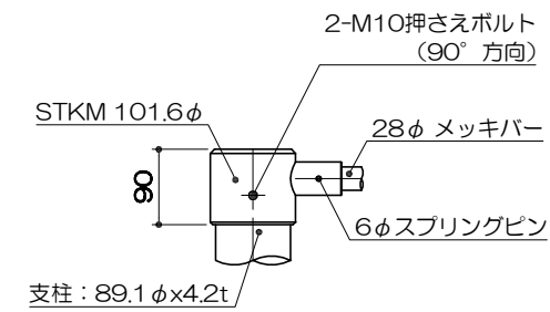
あ部詳細図 S= 1 : 10
