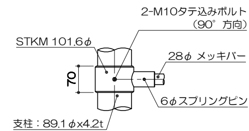
う部詳細図 S= 1 : 10
