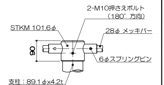
い部詳細図 S= 1 : 10
