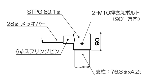
え部詳細図 S= 1 : 10
