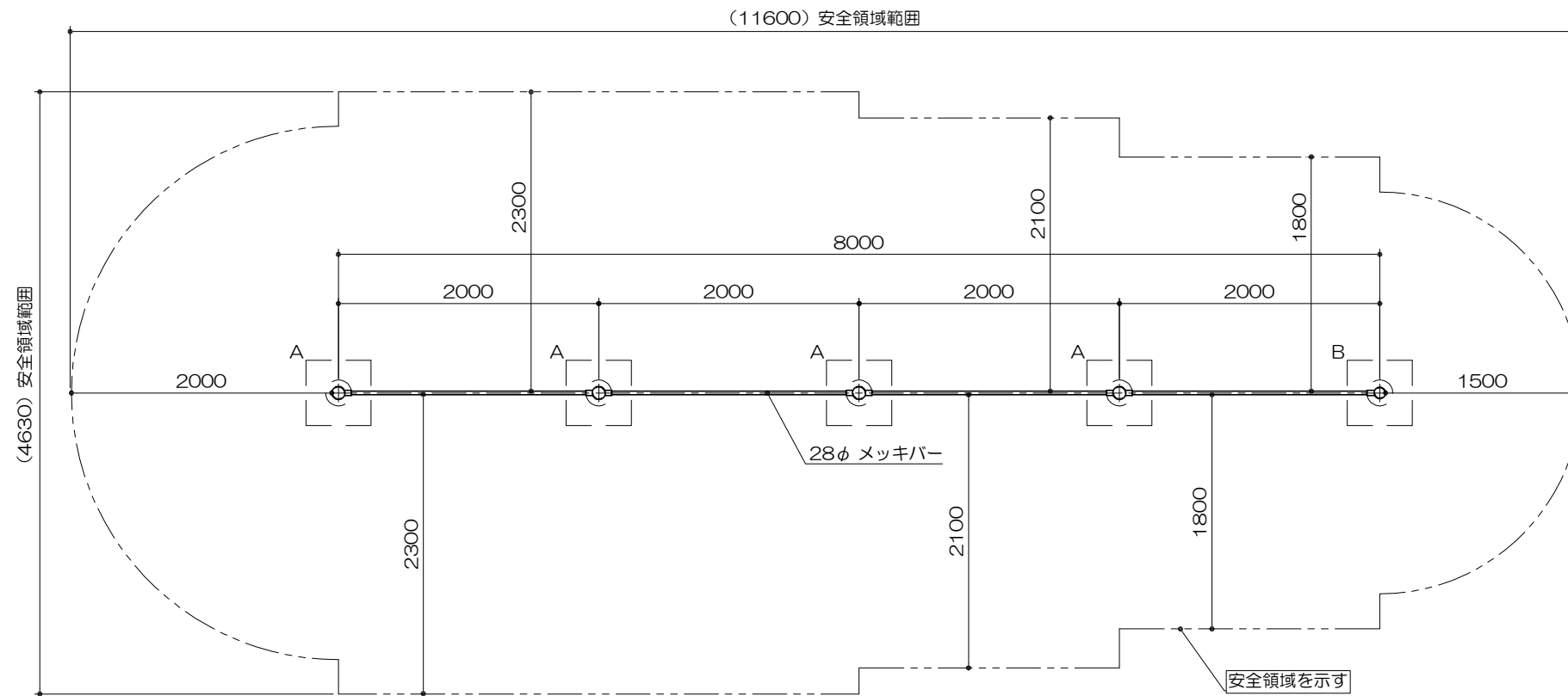
平面図 S= 1 : 50
