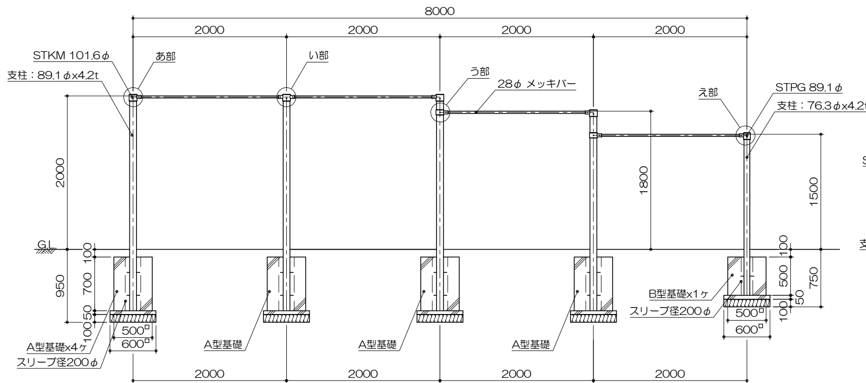
立面図 S= 1 : 50
