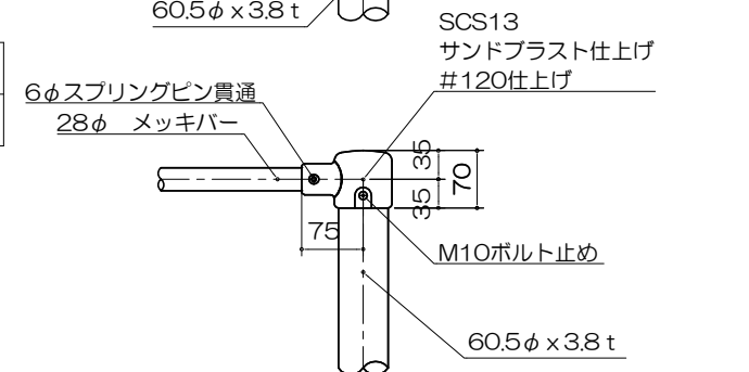
工部詳細図 S= 1 : 10
