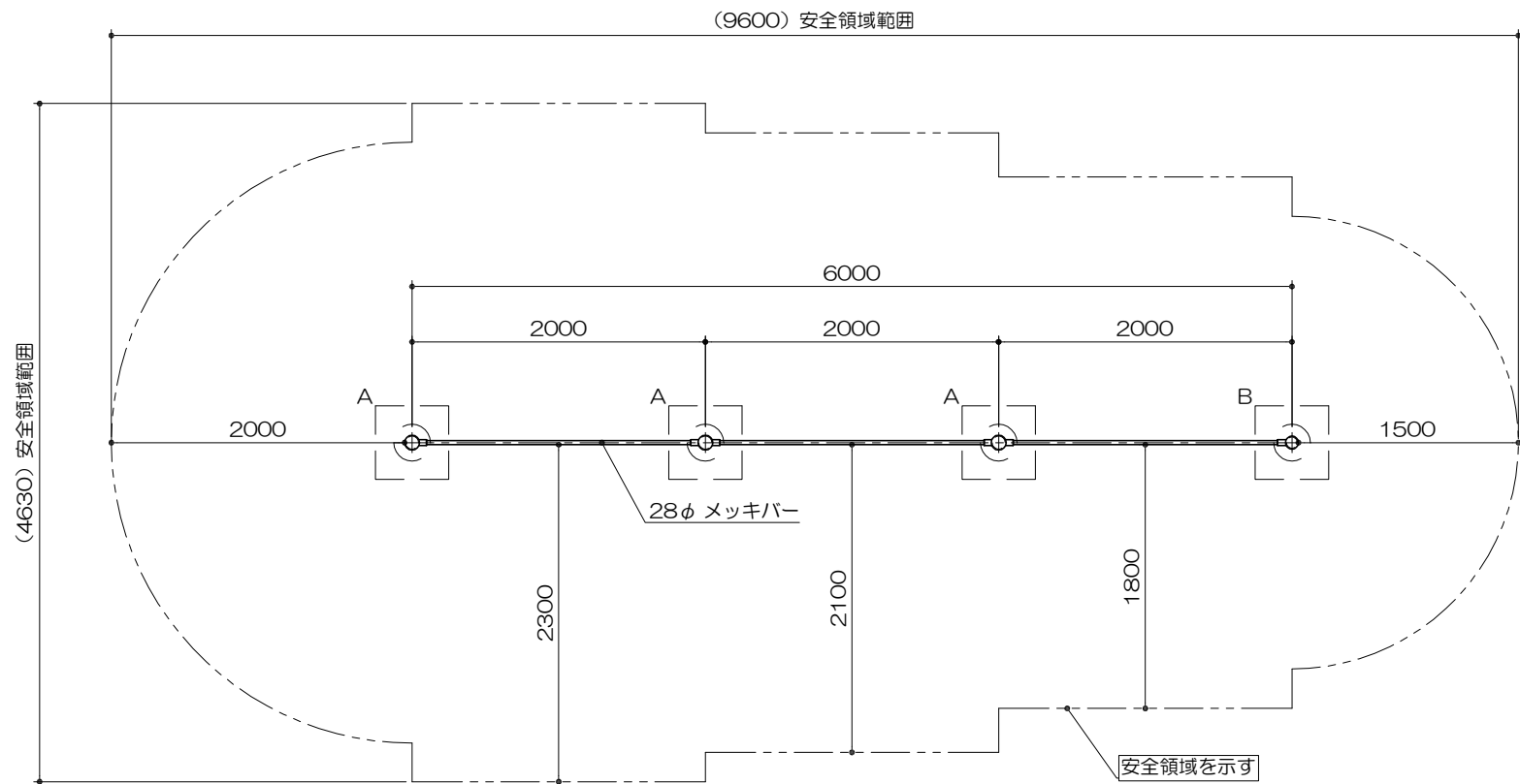
平面図 S= 1 : 50
