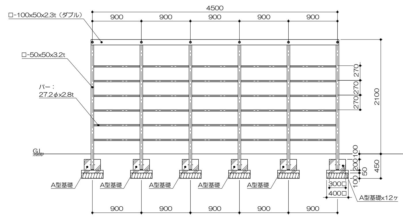
立面図 S= 1 : 40
