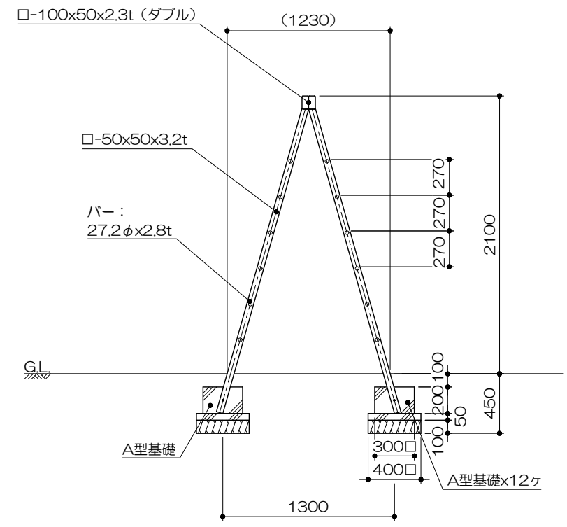
側面図 S= 1 : 40
